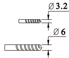
(Ø6 Ø3 2) SVRDLA ZA BUŠILICU DRILL BIT
