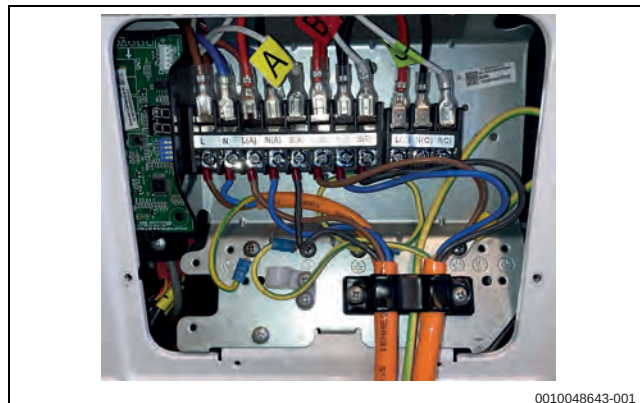
Bild 19 Elektrischer Anschluss
