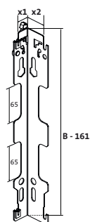
MCW-5 nosač
